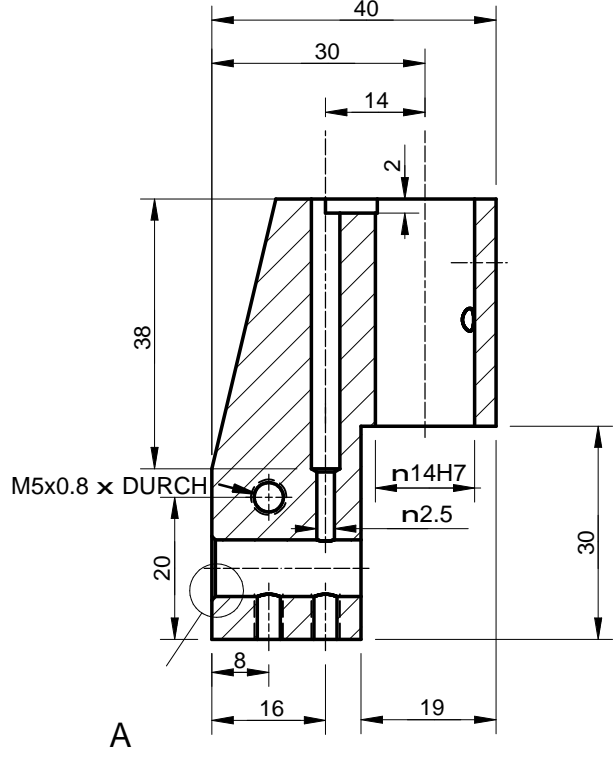
Schnitt C-C
